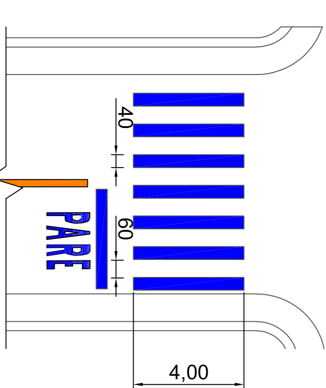
DETALHE 2 - FAIXA DE PEDESTRES
